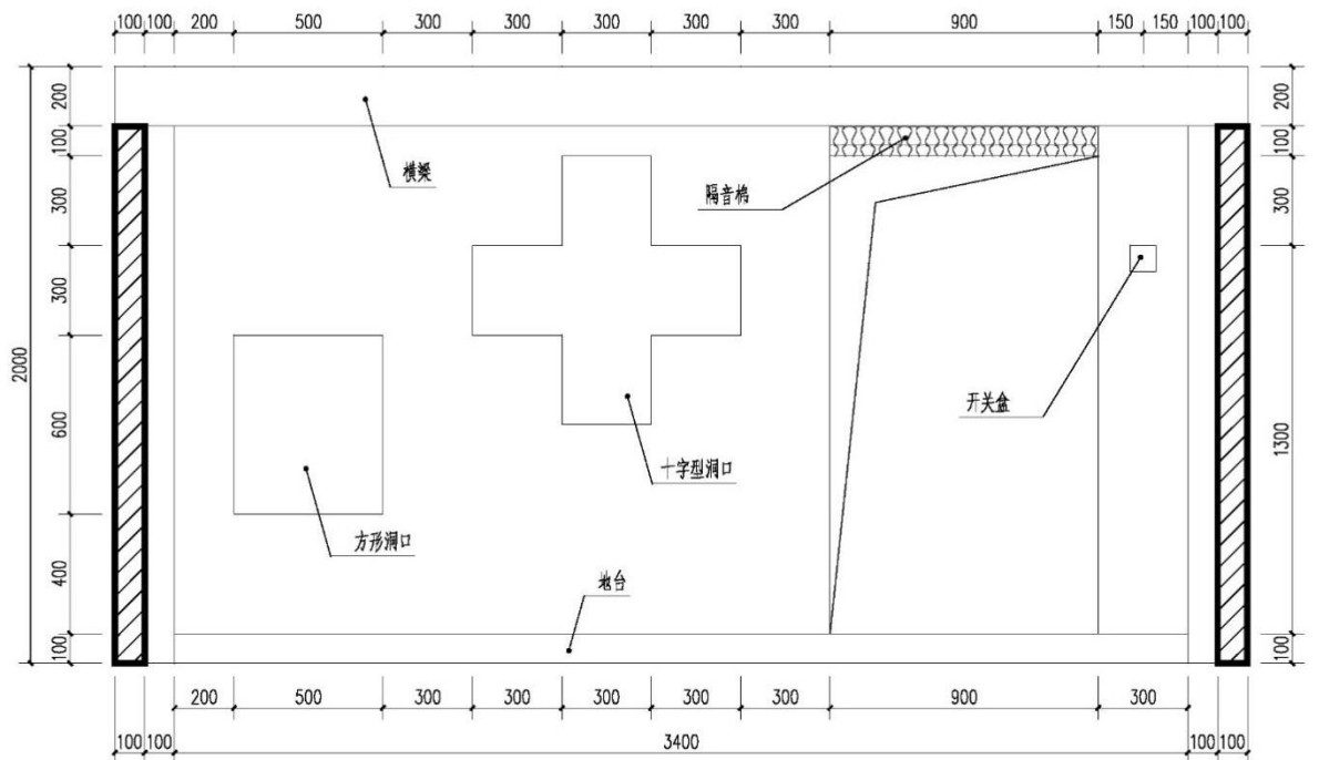
图 4 C 立面图
