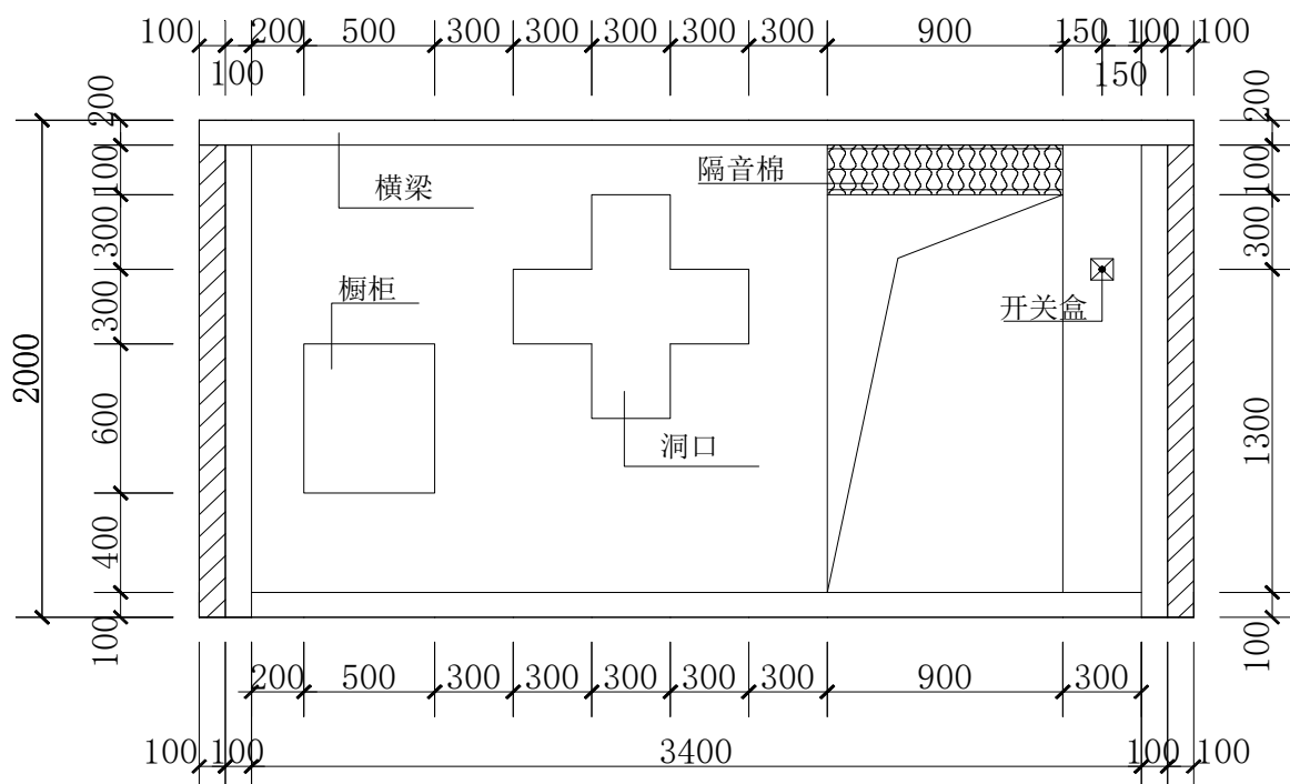
隔墙木作立面图
