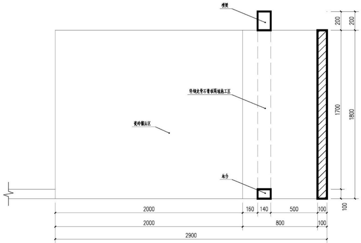
图 3 A 立面图
