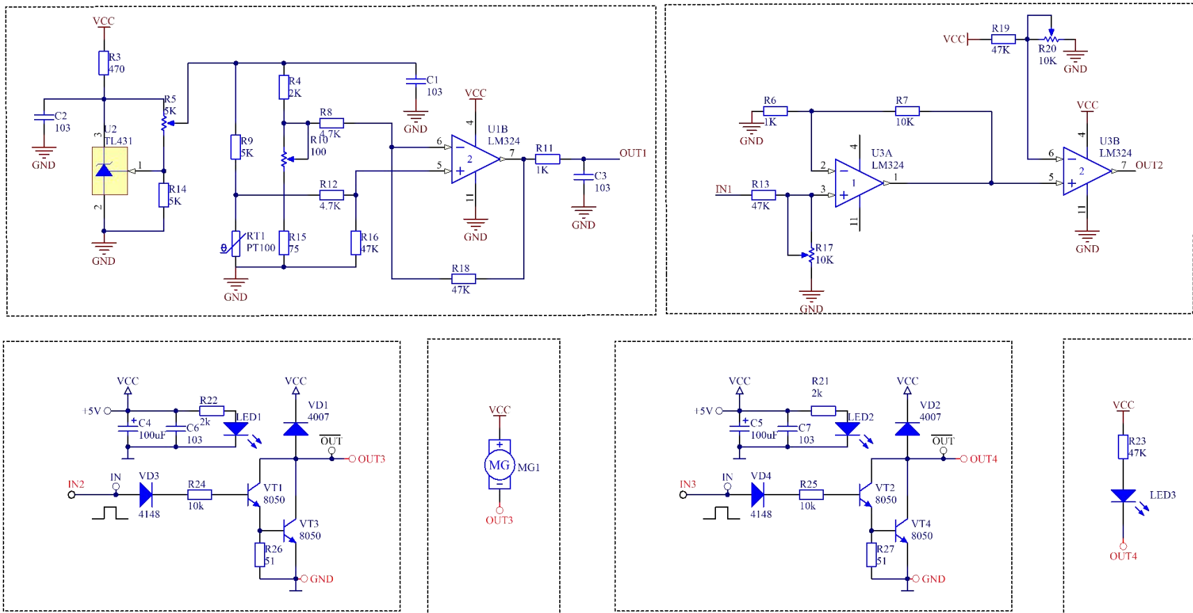
图 4 测温报警系统电路原理图一
