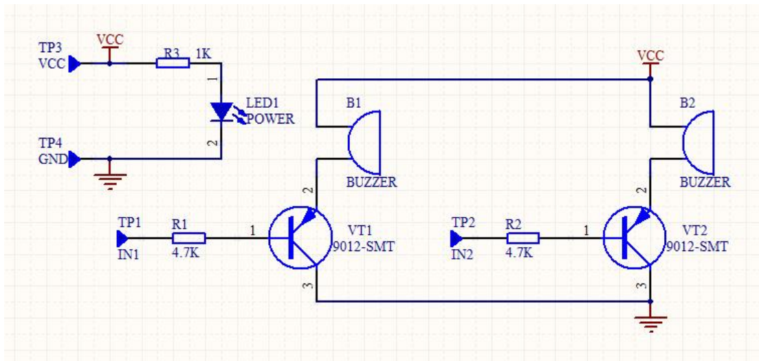
图2 EDM504-蜂鸣器电路原理图
