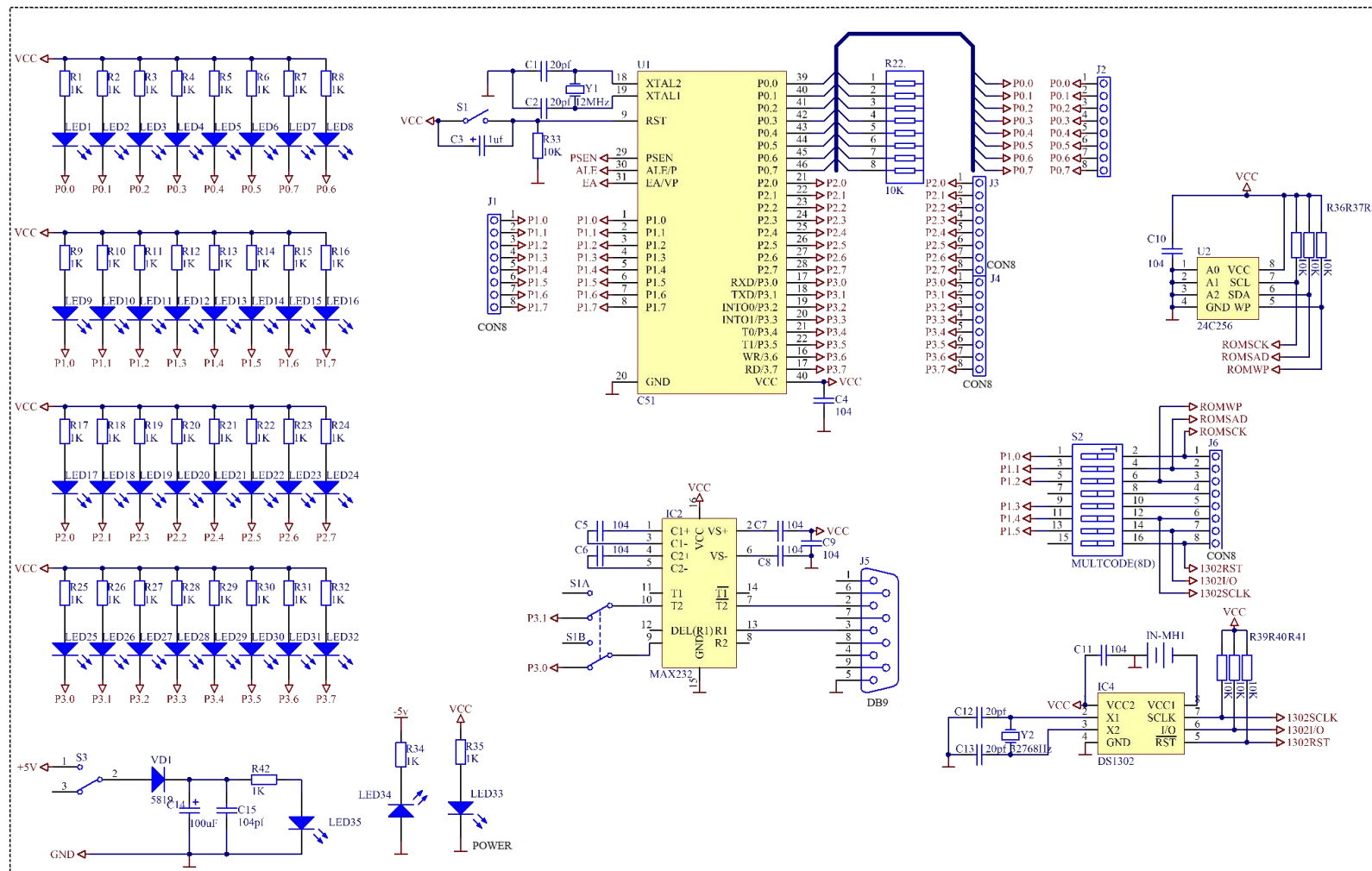
图 5 测温报警系统电路原理图二
