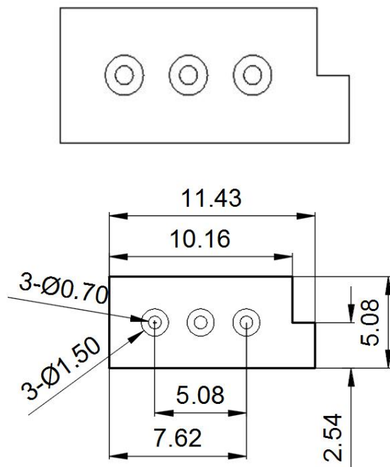
图3 封装尺寸图
